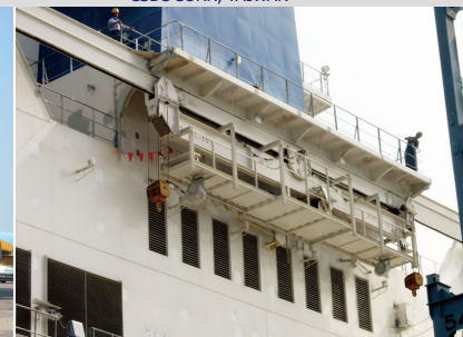
▼ 船舶用(糧食、機艙)吊車/吊桿 台灣國際造船股份有限公司 Provision Crane/Monorail Crane CSBC CORP., TAIWAN
