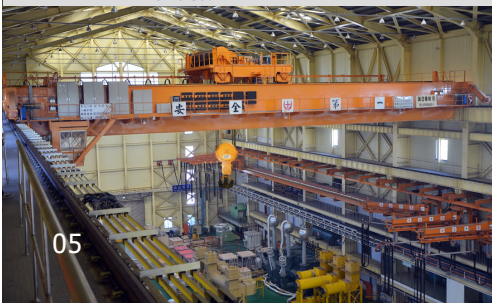
▼ 200/40/5噸架空式天車 大同股份有限公司 200/40/5t Overhead Crane (Twin Hoists) TATUNG CO.
